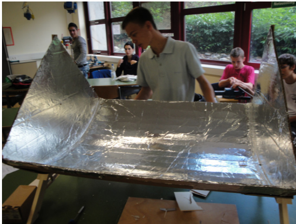
Der fast fertige Solargrill.
